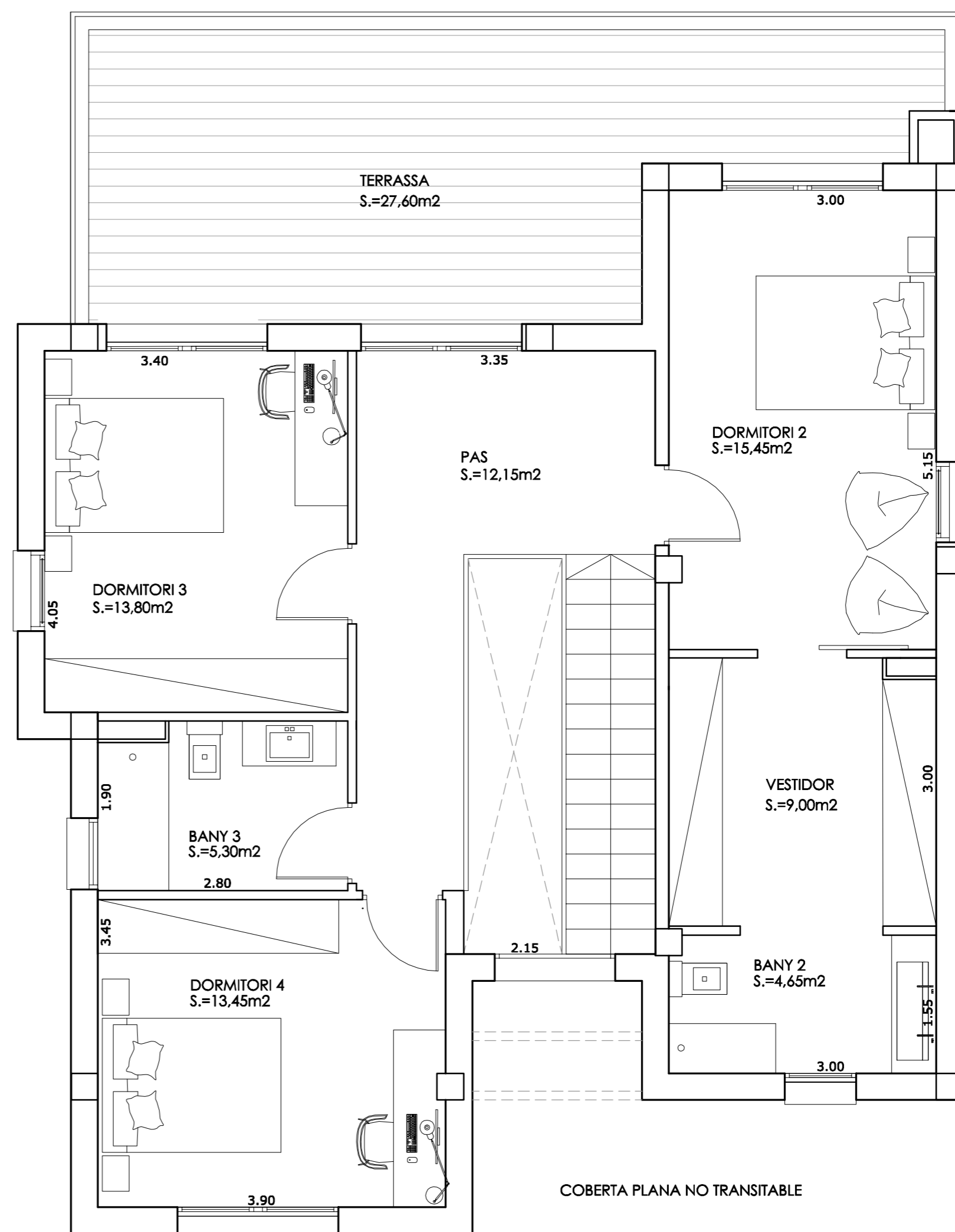
PLANTA 1 SUP CONST. VIV. =100,45m2
